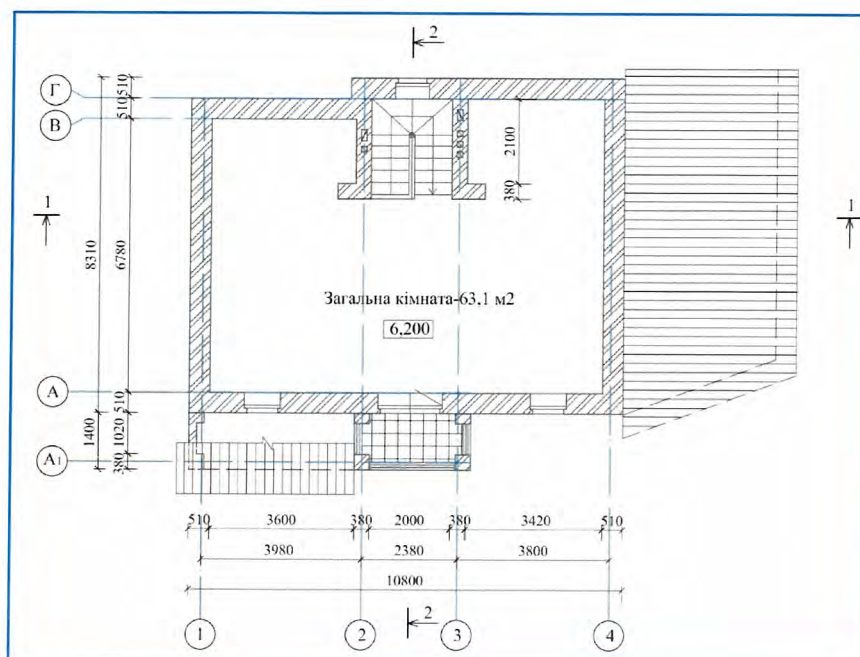
Рисунок 2.4 – План мансардного поверху
