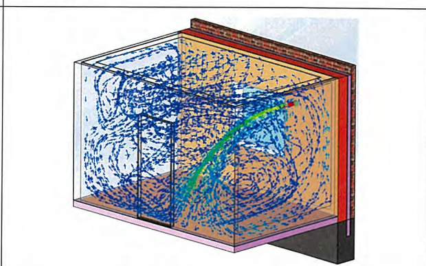
Рисунок 4.21 – Розподіл потоків повітря при стіновій системі опалення
