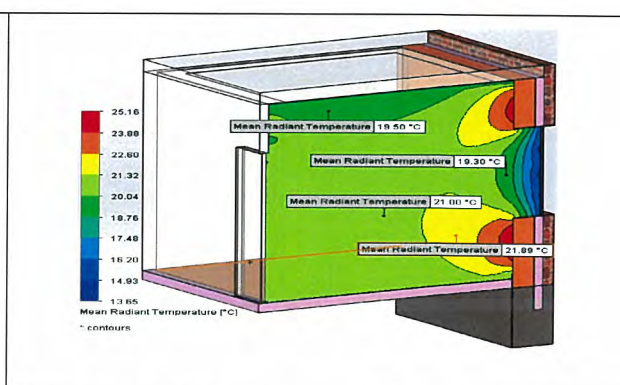
Рисунок 4.19 – Розподіл радіаційної температури при стіновій системі опалення
