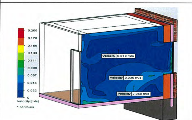
Рисунок 4.20 – Розподіл швидкості повітря при стіновій системі опалення
