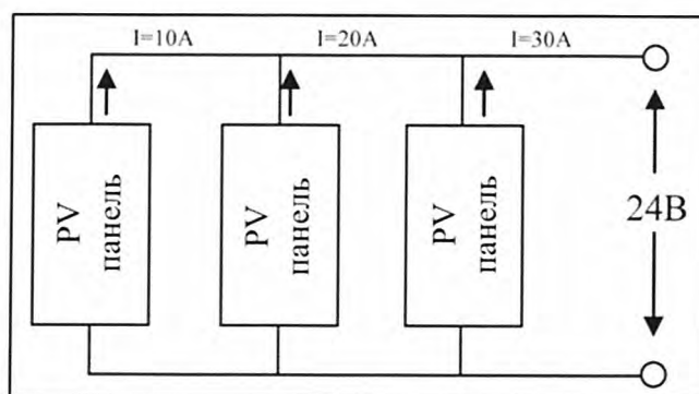
Рисунок 3.5 – Схема підключення трьох панелей
